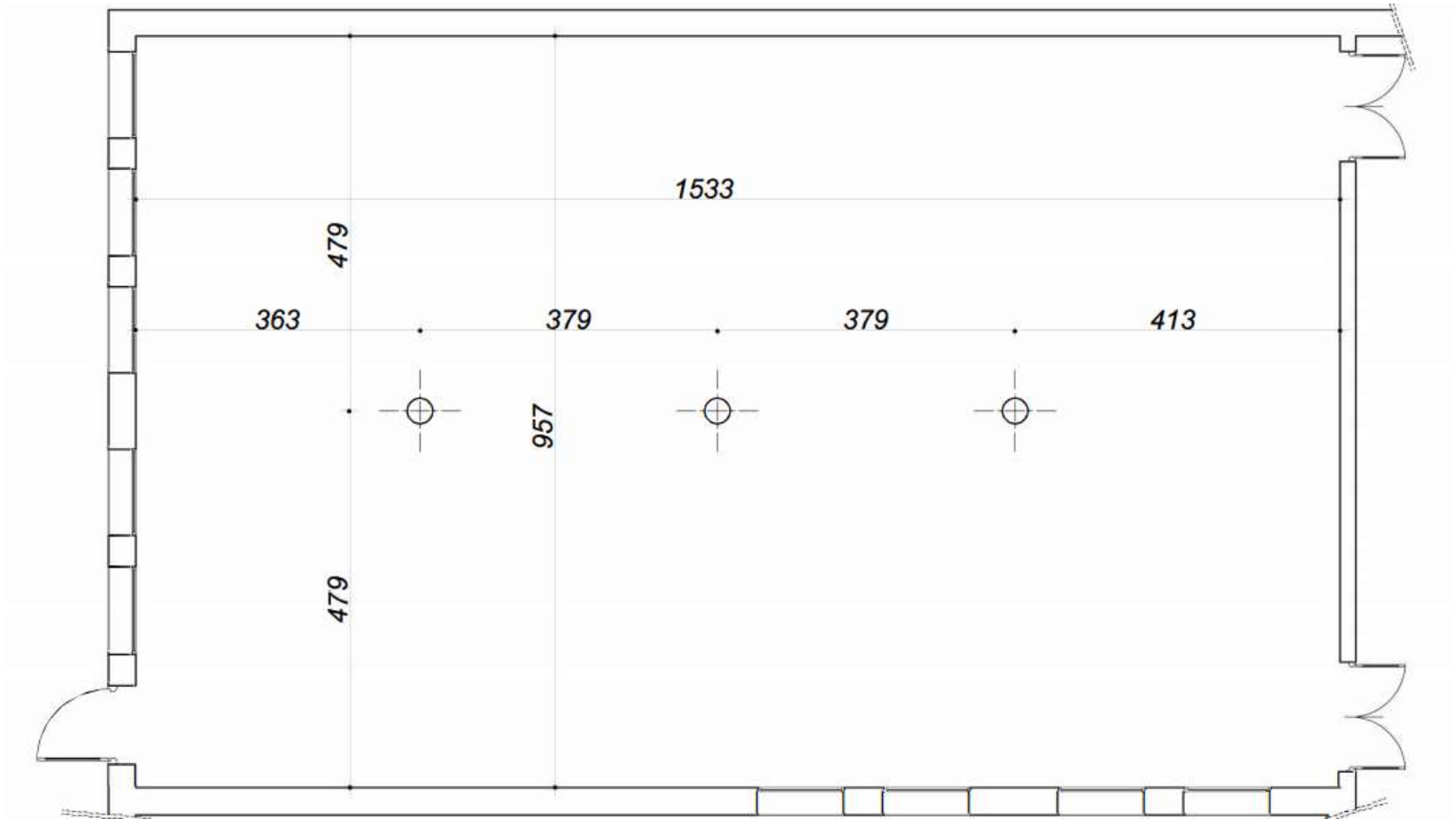
Figure2: Plan de la salle B1 dédiée à une salle polyvalente (pour séminaires, manifestations, formations)
