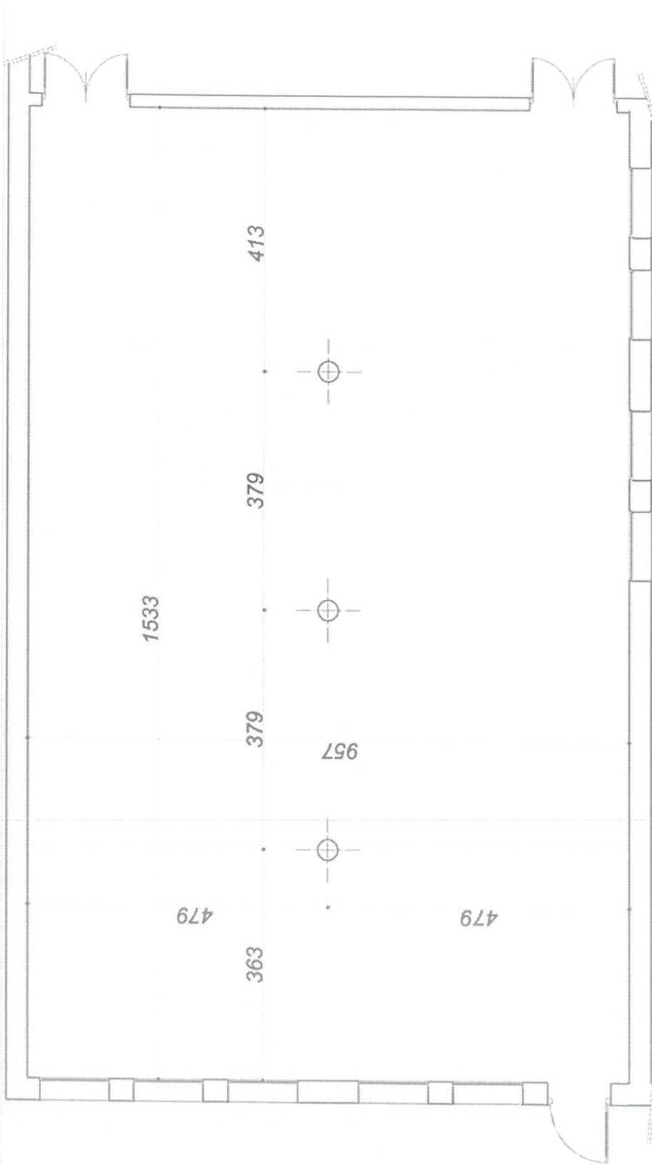
Figure2: Plan de la salle B1 dédiée à une salle polyvalente (pour séminaires, manifestations, formations)
